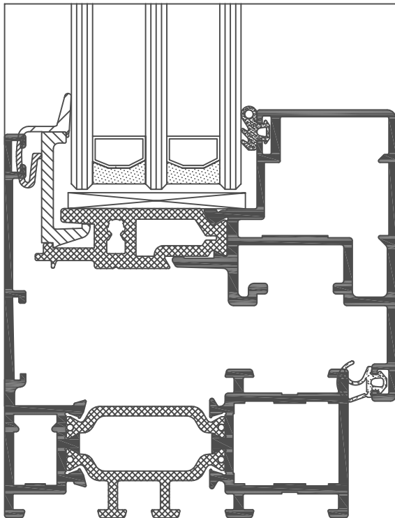
przekrój przez okno EF OC (EF214 + EF222)
