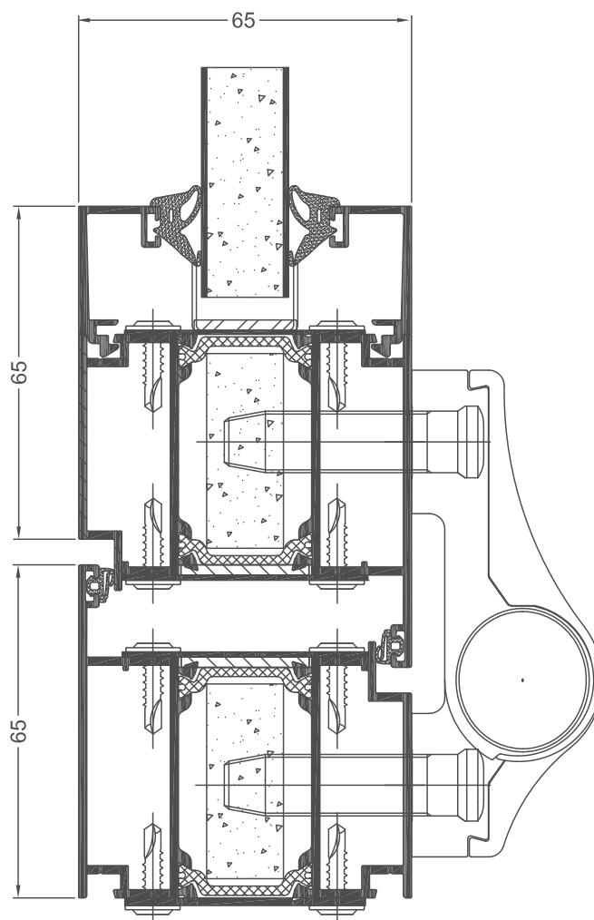
przekrój przez drzwi FR 65 (FR024 + FR024)
